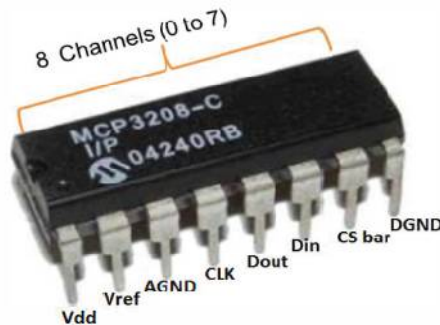
Fig.4: MCP 3208 ADC.
