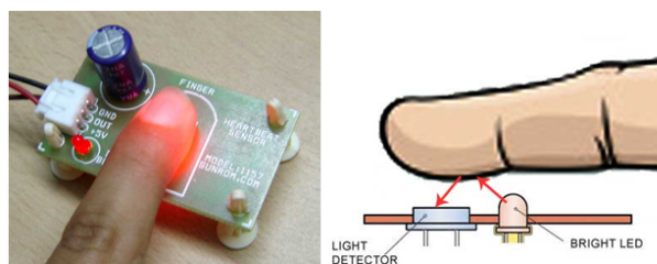
Fig. 1 Heart Beat Sensor
