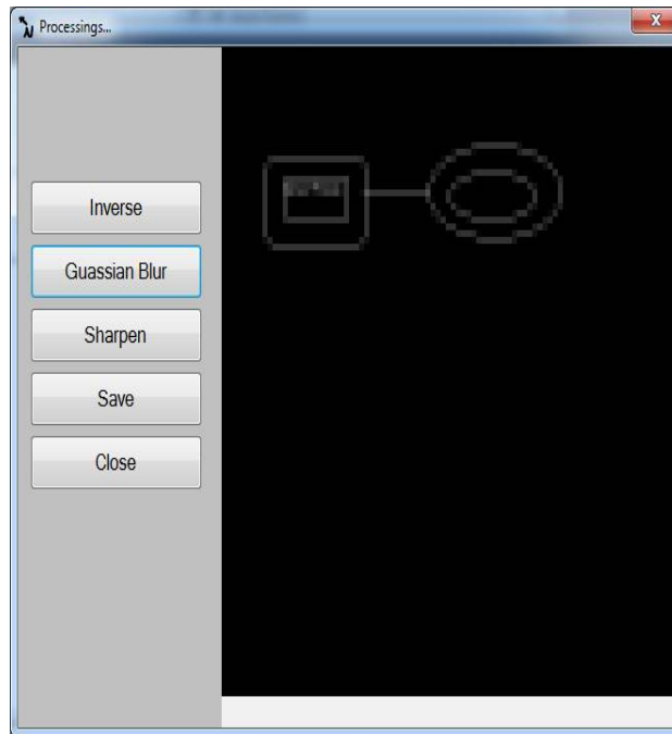
Fig.6. Gaussian Blur
