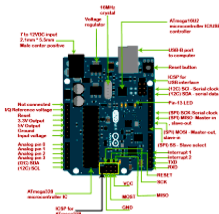
Fig.6 Arduino Uno Board
