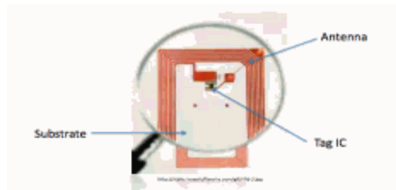
Fig: RFID Tag
